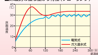
■床暖房の立ち上がり特性(フローリング)
